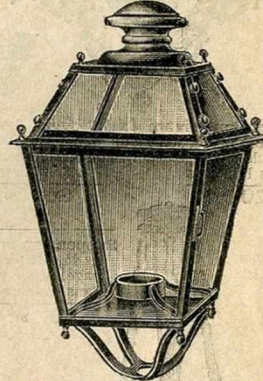
Lanterne de ville ou réverbère pour lampe à pétrole, montée à vis, tôle plombée, bronzée.
